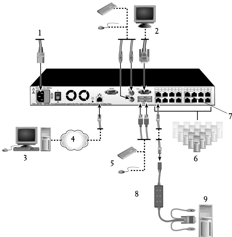
Рис. 2-4. Базовая конфигурация удаленного консольного коммутатора
