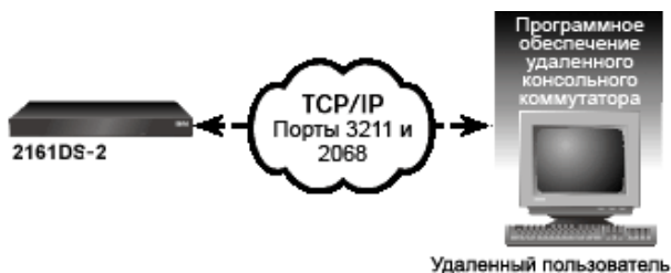
Рис. В-1. Взаимодействие через порты TCP
